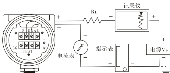
LY37外形变送器外部线路接线图
