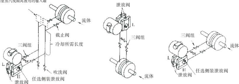
测量蒸汽或隔离液用的输入罐
