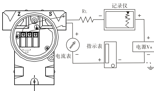
LY36外形变送器外部线路接线图
