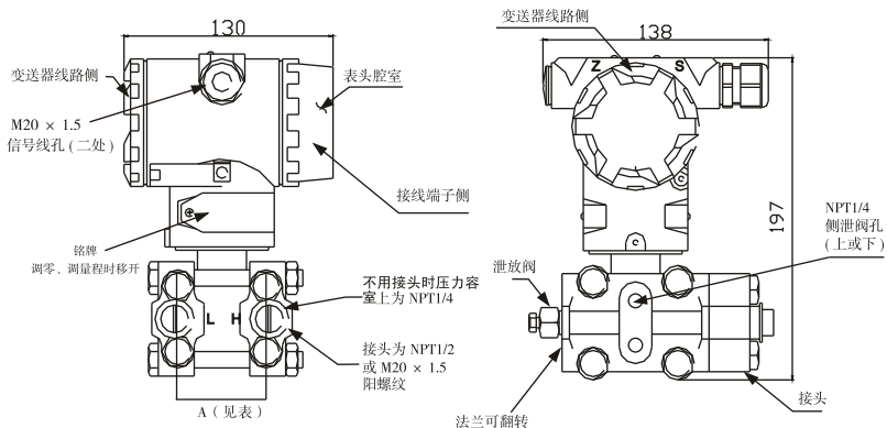
LY36 外形尺寸图
