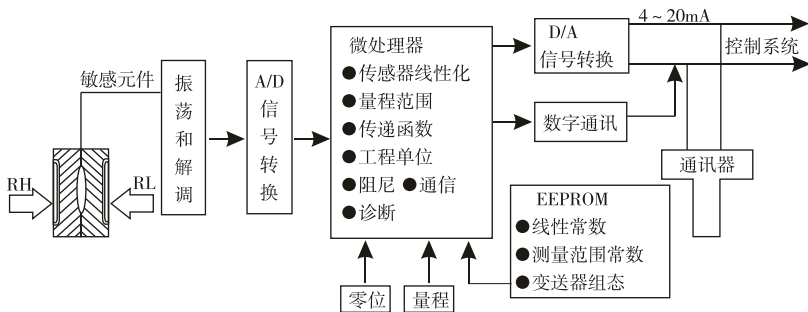
图1-1 工作原理方块图
