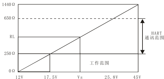
图2-2 负载特性图
