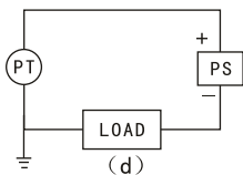
图1-3接地时快速采样计算机在精度上的影响
