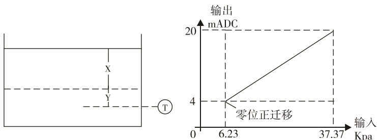
图4-2 开口容器液体测量举例
