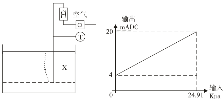
图4-4 吹气法测量液位举例
