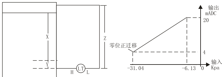
图4-3 密闭容器导压连接测量举例
