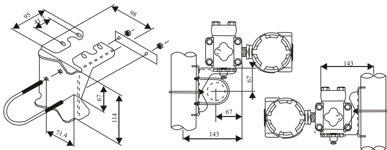
管装弯支架 B1
