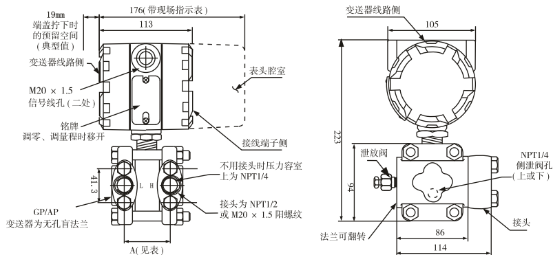
LY37 外形尺寸图
