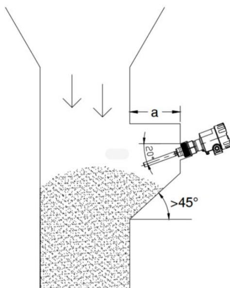
图3 壁龛式安装示意图
