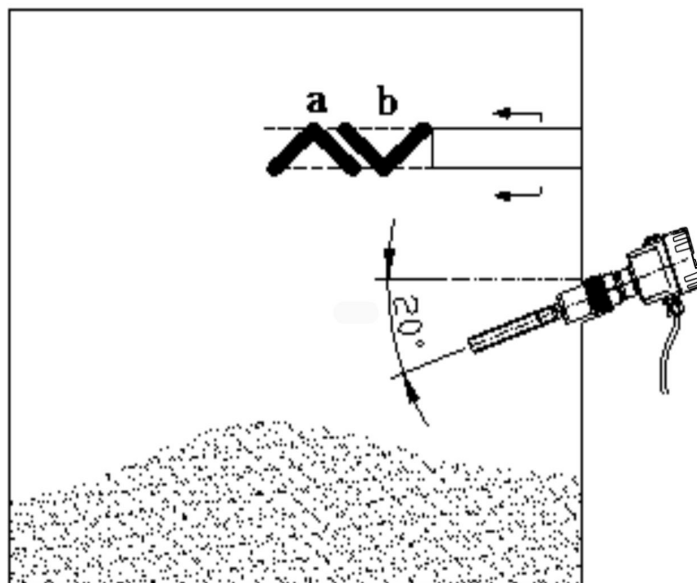
图 2 挡板式安装示意图
