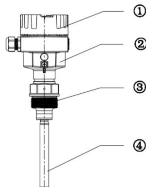
图 1 LSF04 整体结构图
