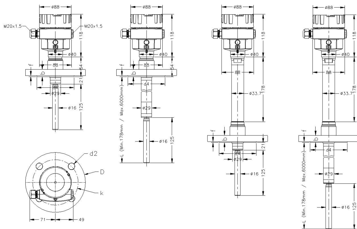
LSF04-法兰
