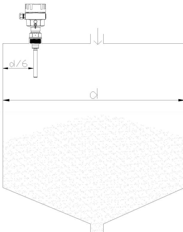
图4 垂直安装示意图
