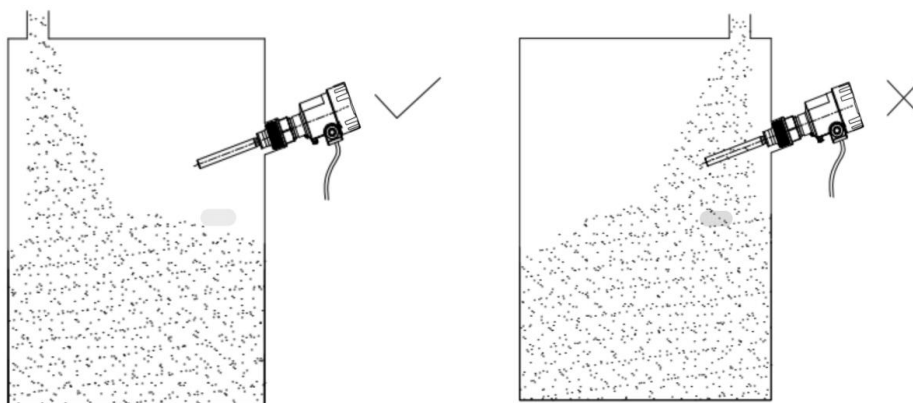
图 5 避开入料口的安装示意图
