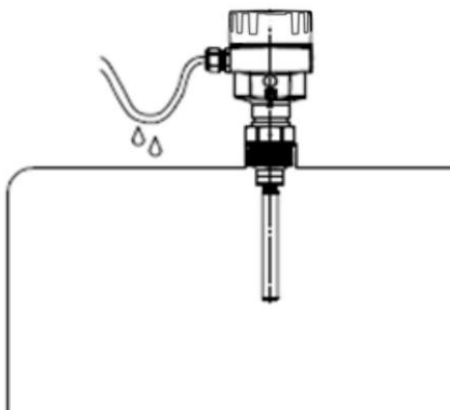
图 6 防潮安装
